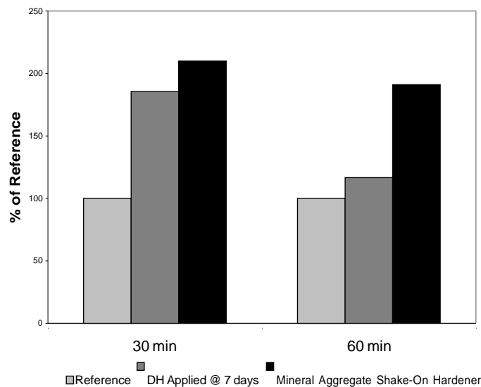
EUCO DIAMOND HARD ASTM C 779 slijtvastheidsresultaten @ 28 dagen
