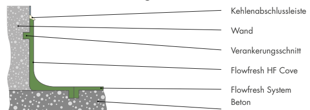
Boden-Wand-Anbindung
