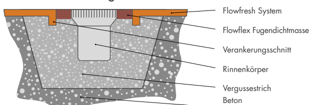
Bodenentwässerung
