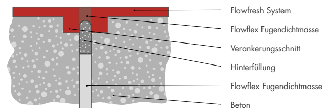
(Dehnungs-) Bewegungsfuge
