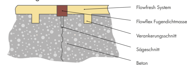
Scheinfuge
