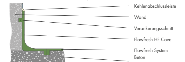
Boden-Wand-Anbindung
