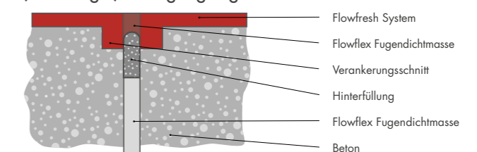
(Dehnungs-) Bewegungsfuge
