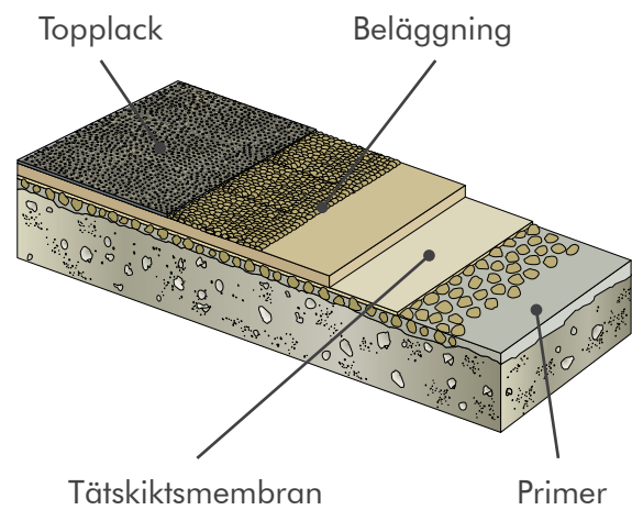
Yttre däck
